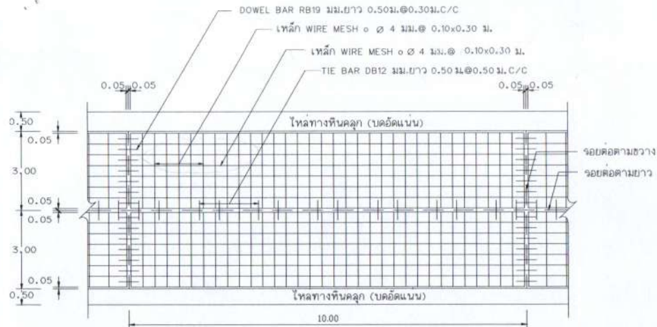
รูปแบบลวดจางรอกอนกรีตเสริมเหล็ก
