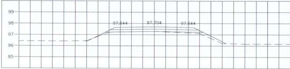
STA. 0+950.000 NGL = 97.305
