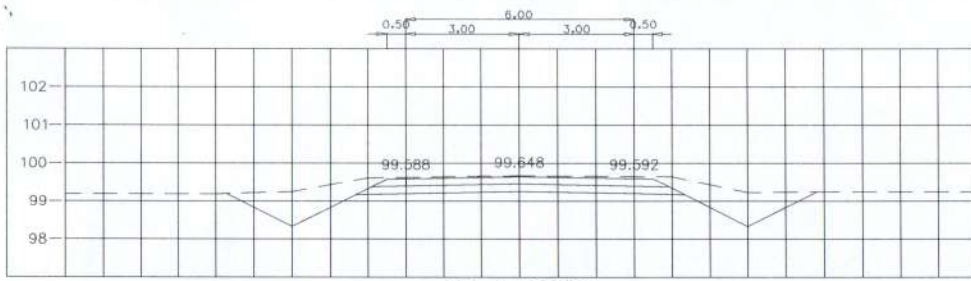
STA. 0+100.000 NGL = 99.670
