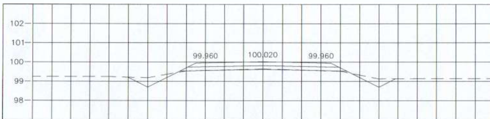
STA. 0+250.000 NGL = 99.640
