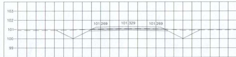
STA. 0+800.000 NGL = 101.075
