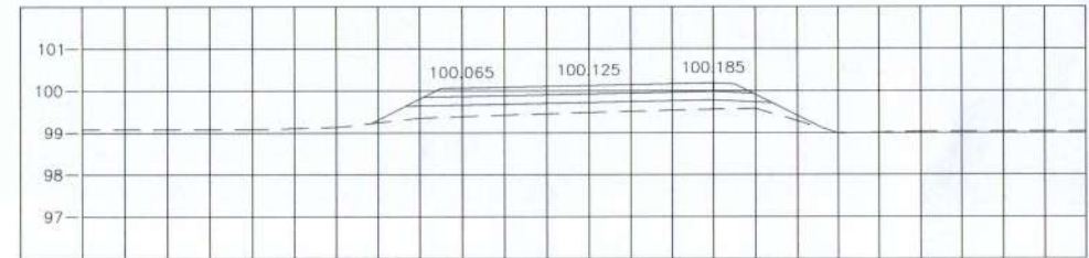
STA. 0+375.000 NGL = 99.490
