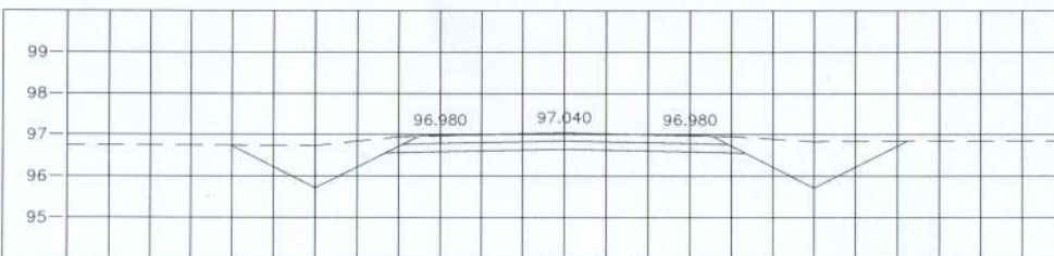
STA. 0+000.000 NGL = 97.040
