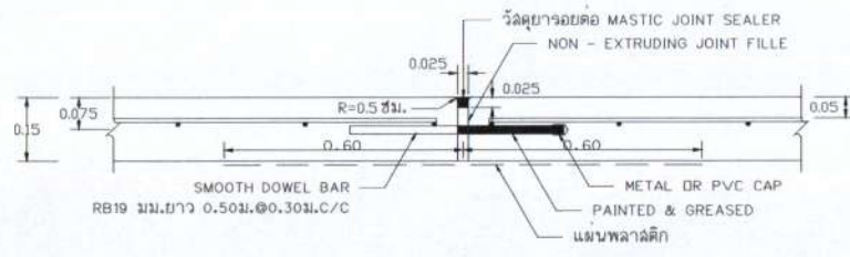
ขยายรอยต่อ EXPANSION JOINT
