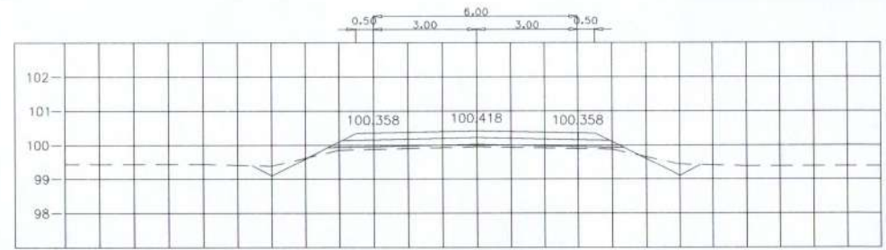
STA. 0+425.000 NGL = 99.950
