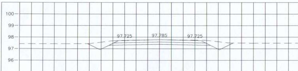
STA. 0+025.000 NGL = 97.780
