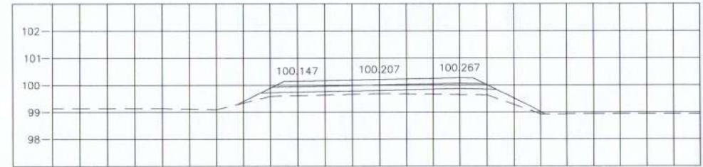
STA. 0+400.000 NGL = 99.680
