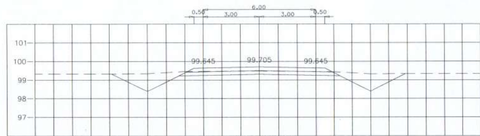
STA. 0+875.000 NGL = 99.485
