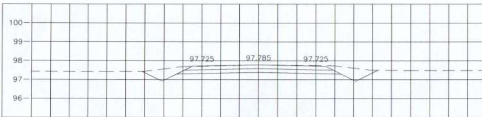
STA. 0+025.000 NGL = 97.780
