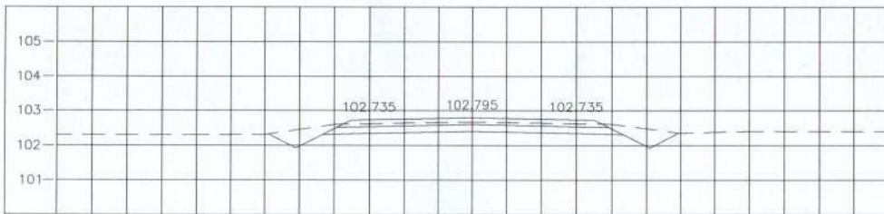
STA. 0+675.000 NGL = 102.670
