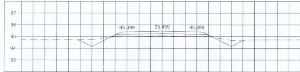
STA. 1+025.000 NGL = 95.035
