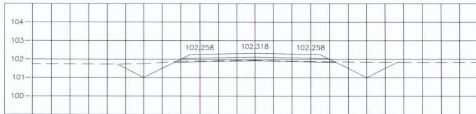
STA. 0+750.000 NGL = 101.935
