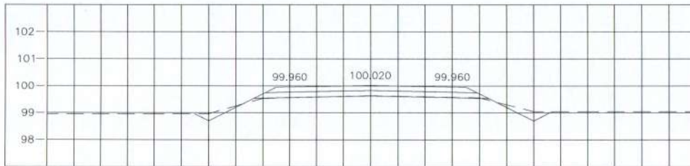
STA. 0+275.000 NGL = 99.630
