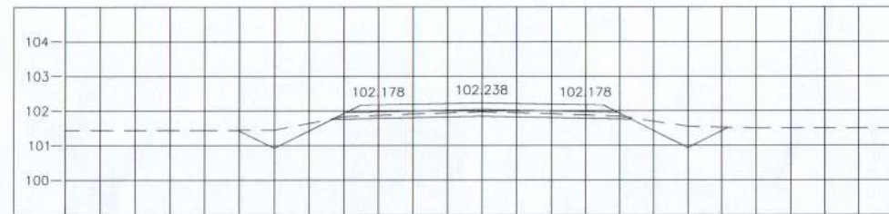
STA. 0+575.000 NGL = 101.975
