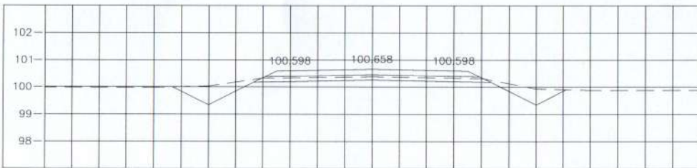
STA. 0+450.000 NGL = 100.380
