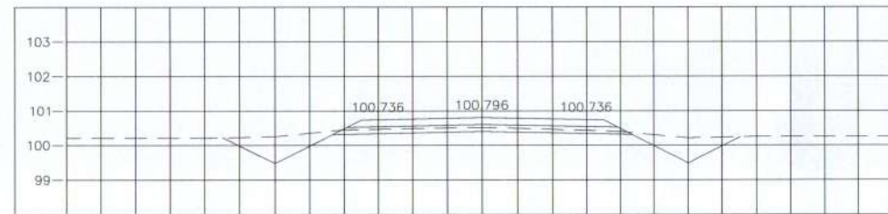
STA. 0+825.000 NGL = 100.515
