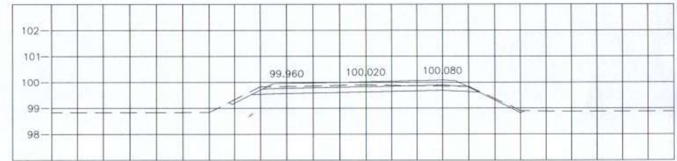
STA. 0+150.000 NGL = 98.890
