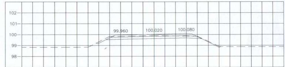
STA. 0+150.000 NGL = 99.890
