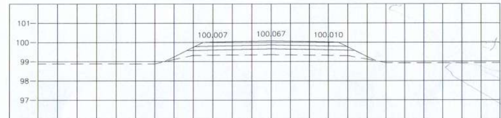
STA. 0+350.000 NGL = 99.360
