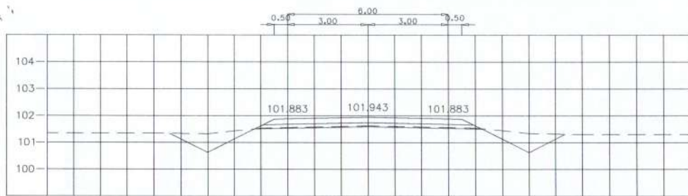
STA. 0+550.000 NGL = 101.625
