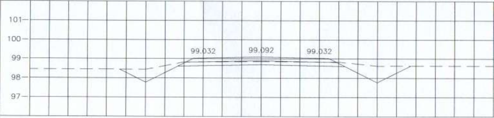
STA. 0+900.000 NGL = 98.855
