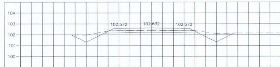
STA. 0+625.000 NGL = 102.395
