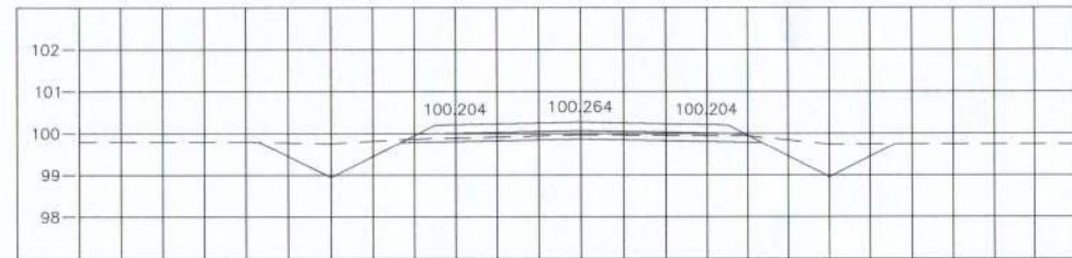
STA. 0+850.000 NGL = 99.965
