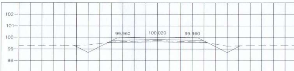
STA. 0+225.000 NGL = 99.730
