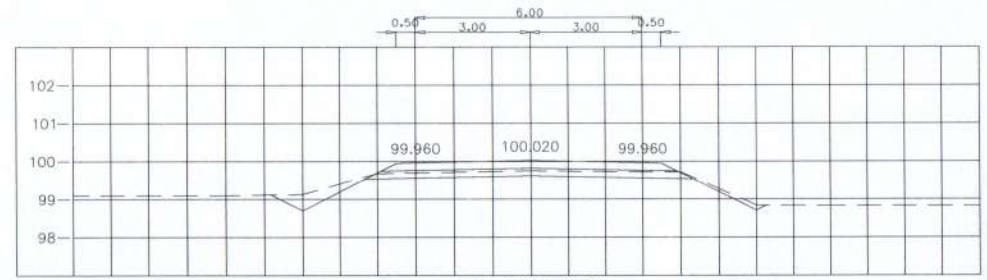
STA. 0+200.000 NGL = 99.750
