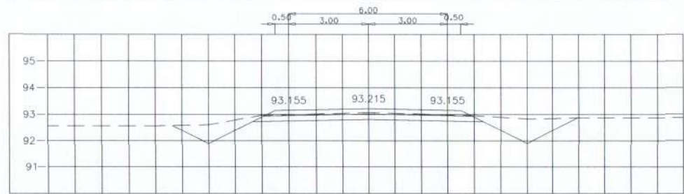
STA. 1+100.000 NGL = 93.065
