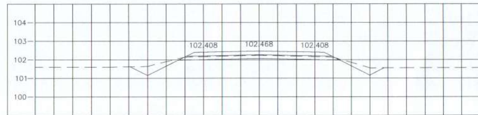
STA. 0+600.000 NGL = 102.245
