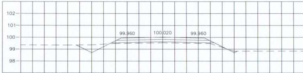
STA. 0+300.000 NGL = 99.530
