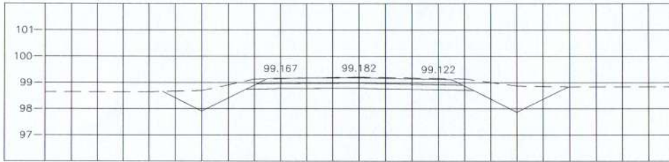
STA. 0+075.000 NGL = 99.210
