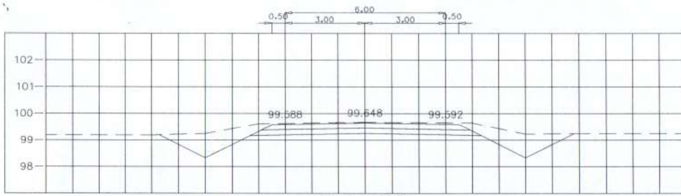
STA. 0+100.000 NGL = 99.670
