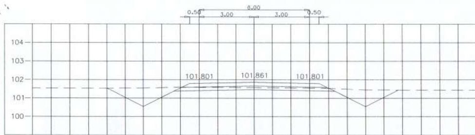
STA. 0+775.000 NGL = 101.575
