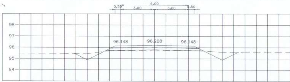
STA. 1+000.000 NGL = 95.775
