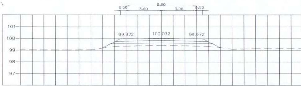
STA. 0+325.000 NGL = 99.430
