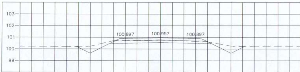
STA. 0+475.000 NGL = 100.780
