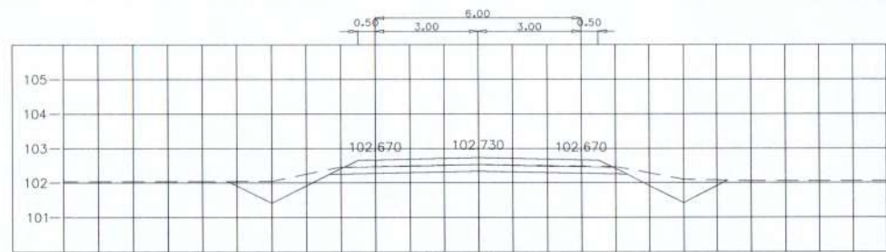
STA. 0+650.000 NGL = 102.535
