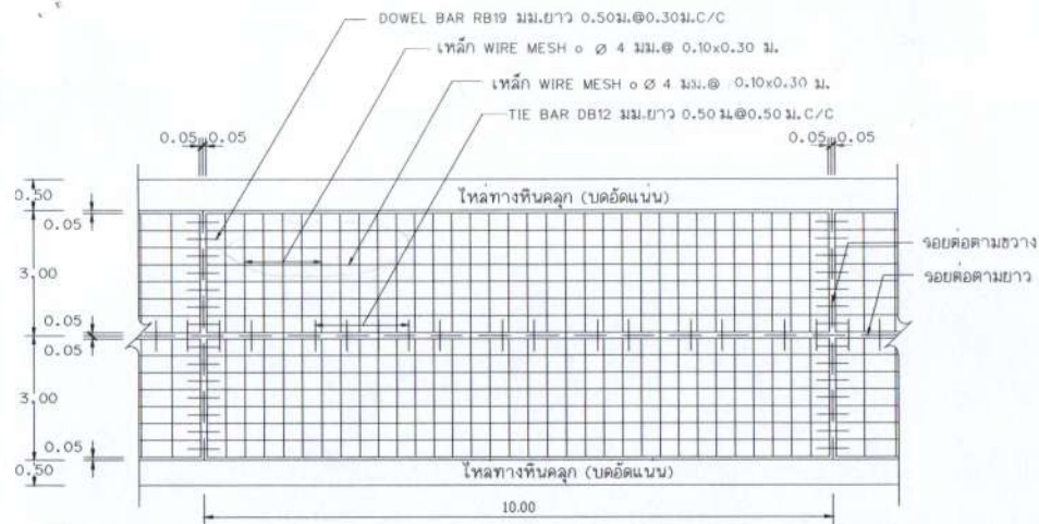
รูปแบบผนังจากรคอนกรีตเสริมเหล็ก
