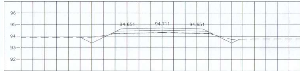
STA. 1+050.000 NGL = 94.335
