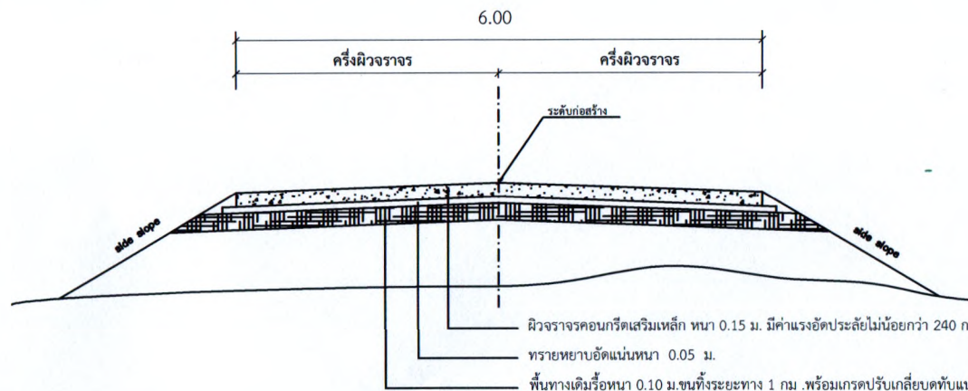
รูปตัดโครงสร้างถนน คสล.
